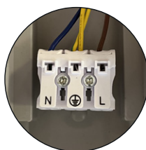
Connecteurs rapides repiquables
